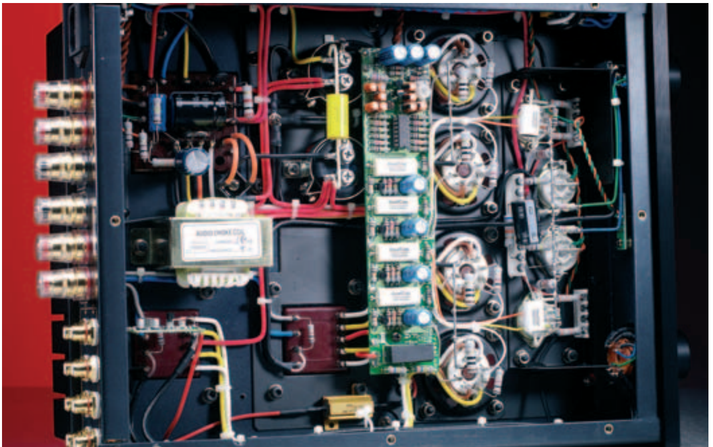
PROLOGUE ONE & TWO: In China sauber handverdrahtet, die Ruhestromregelungs-Platine (Mitte) bekamen sie in Holland dazu.
